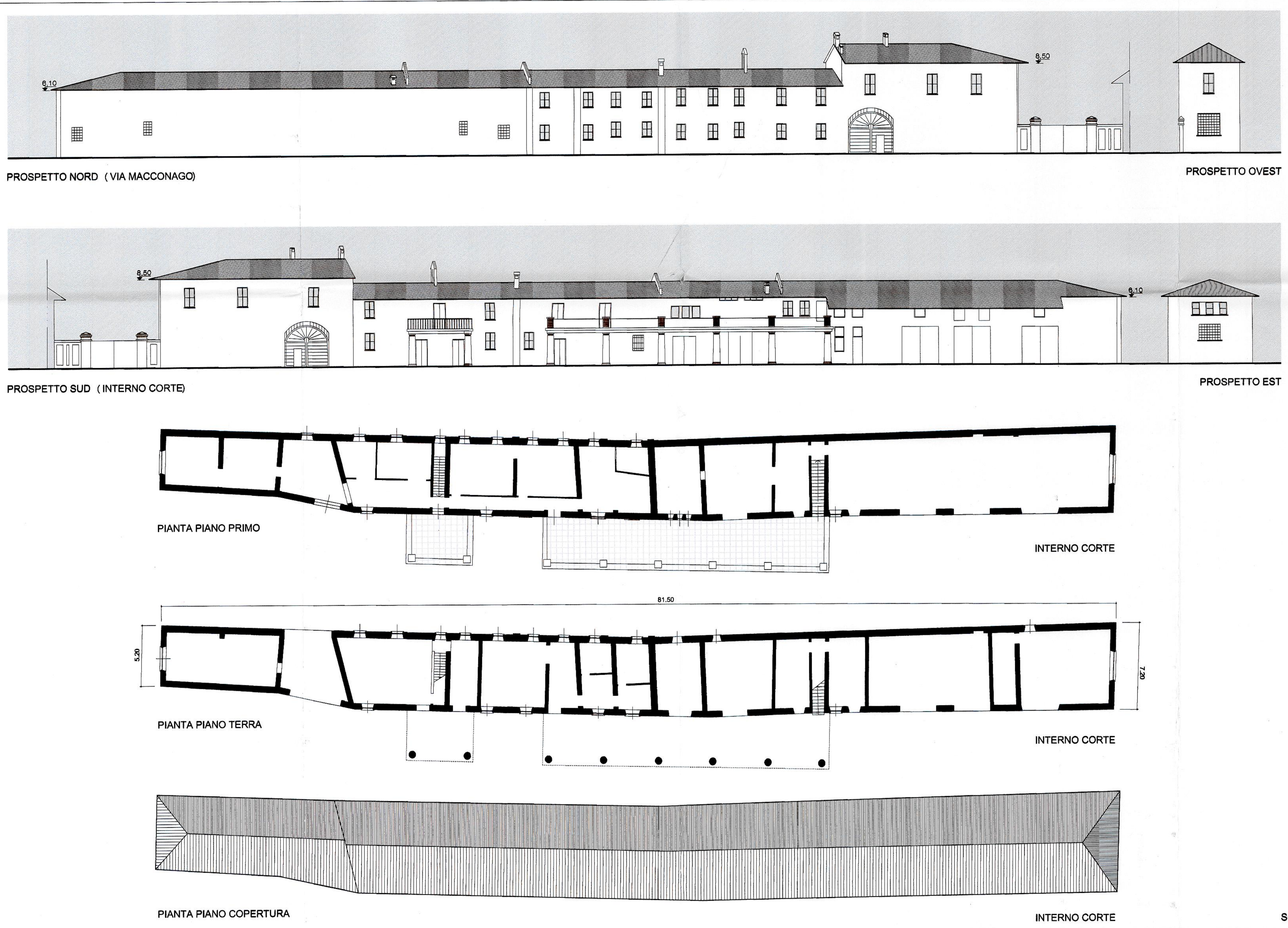
PIANTE - PROSPETTI EDIFICIO PADRONALE OGGETTO DI RISTRUTTURAZIONE EDILIZIA
