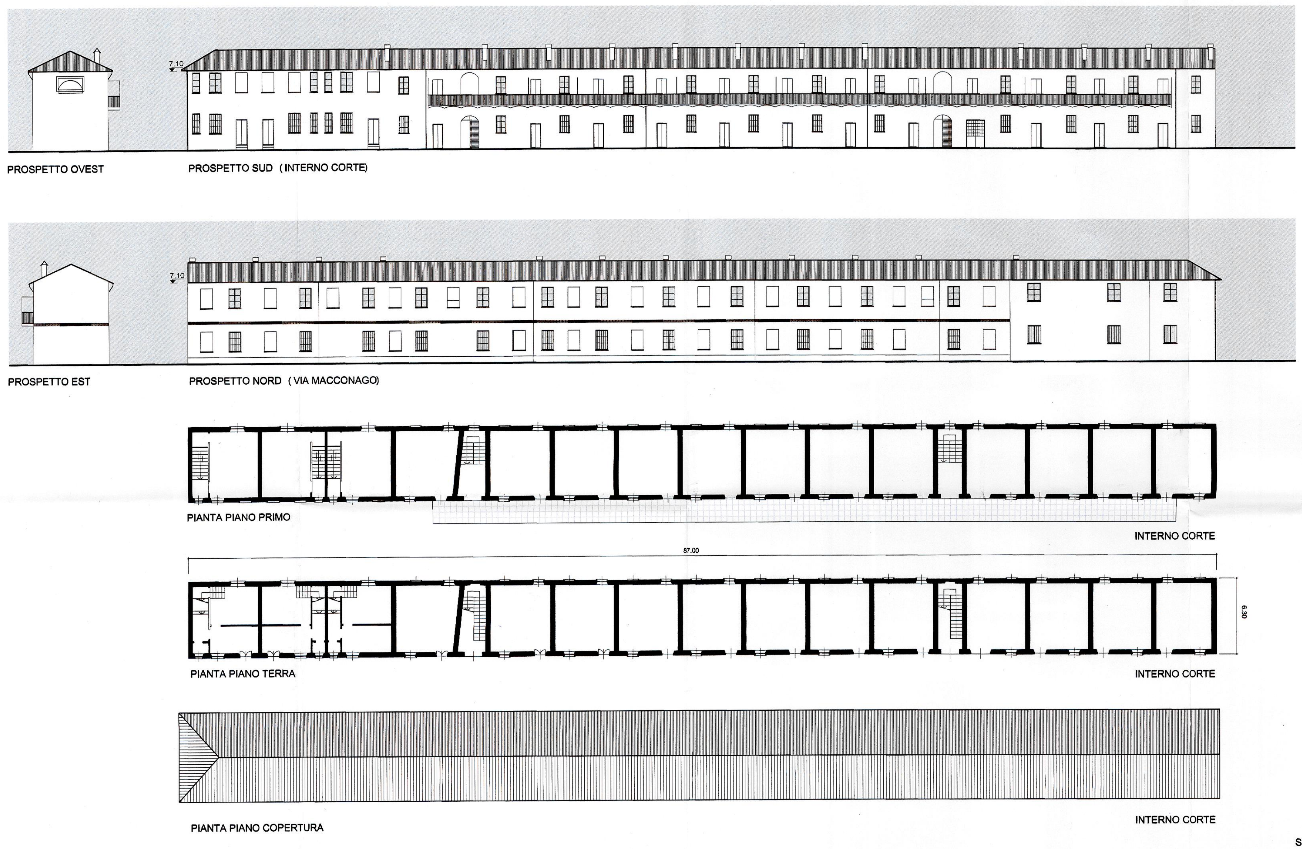
PIANTE - PROSPETTI EDIFICIO SALARIATI OGGETTO DI RISTRUTTURAZIONE EDILIZIA
