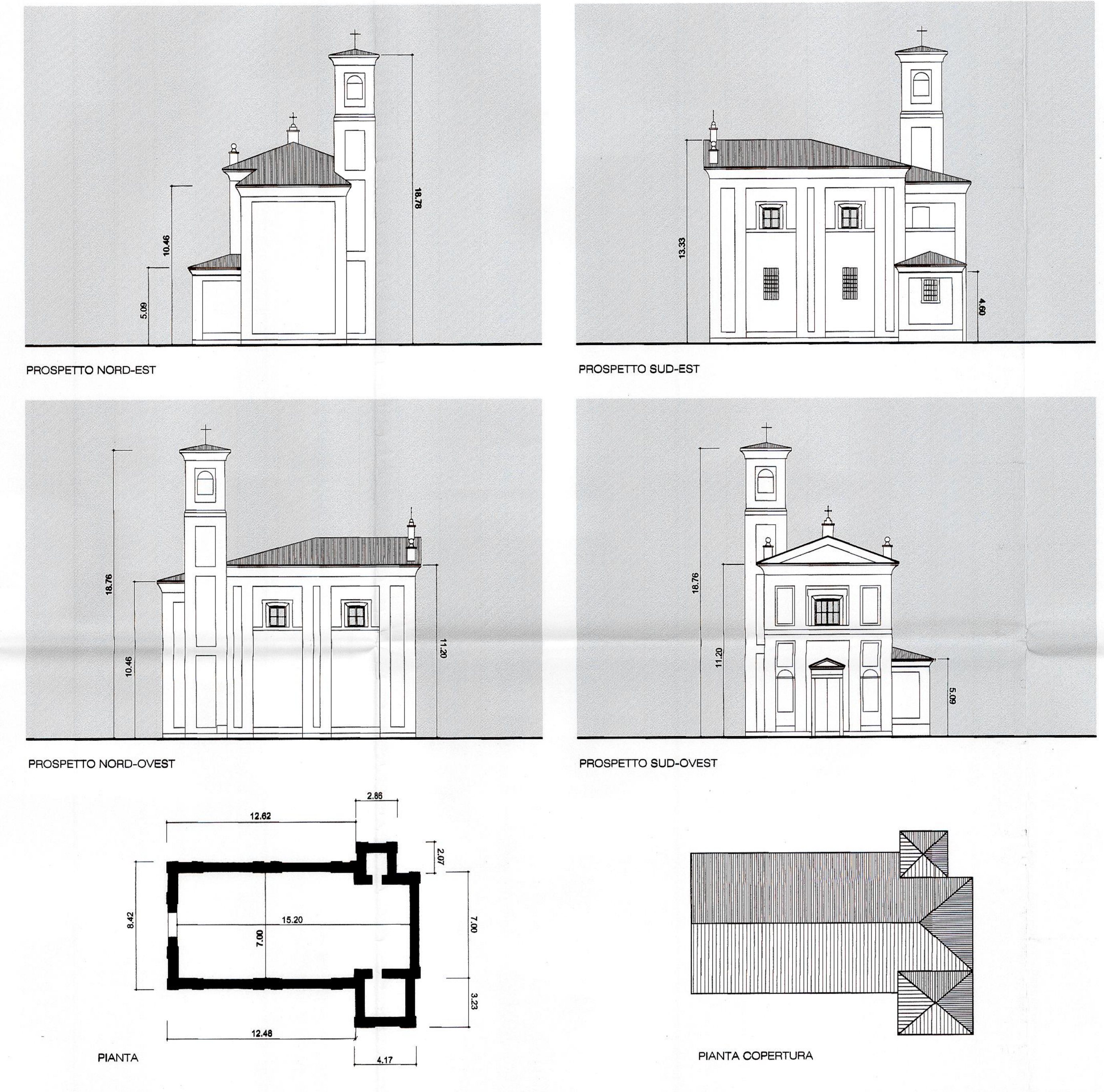
PIANTE PROSPETTI E IMMAGINI FOTOGRAFICHE EX CHIESETTA DI SAN CARLO OGGETTO DI RESTAURO
